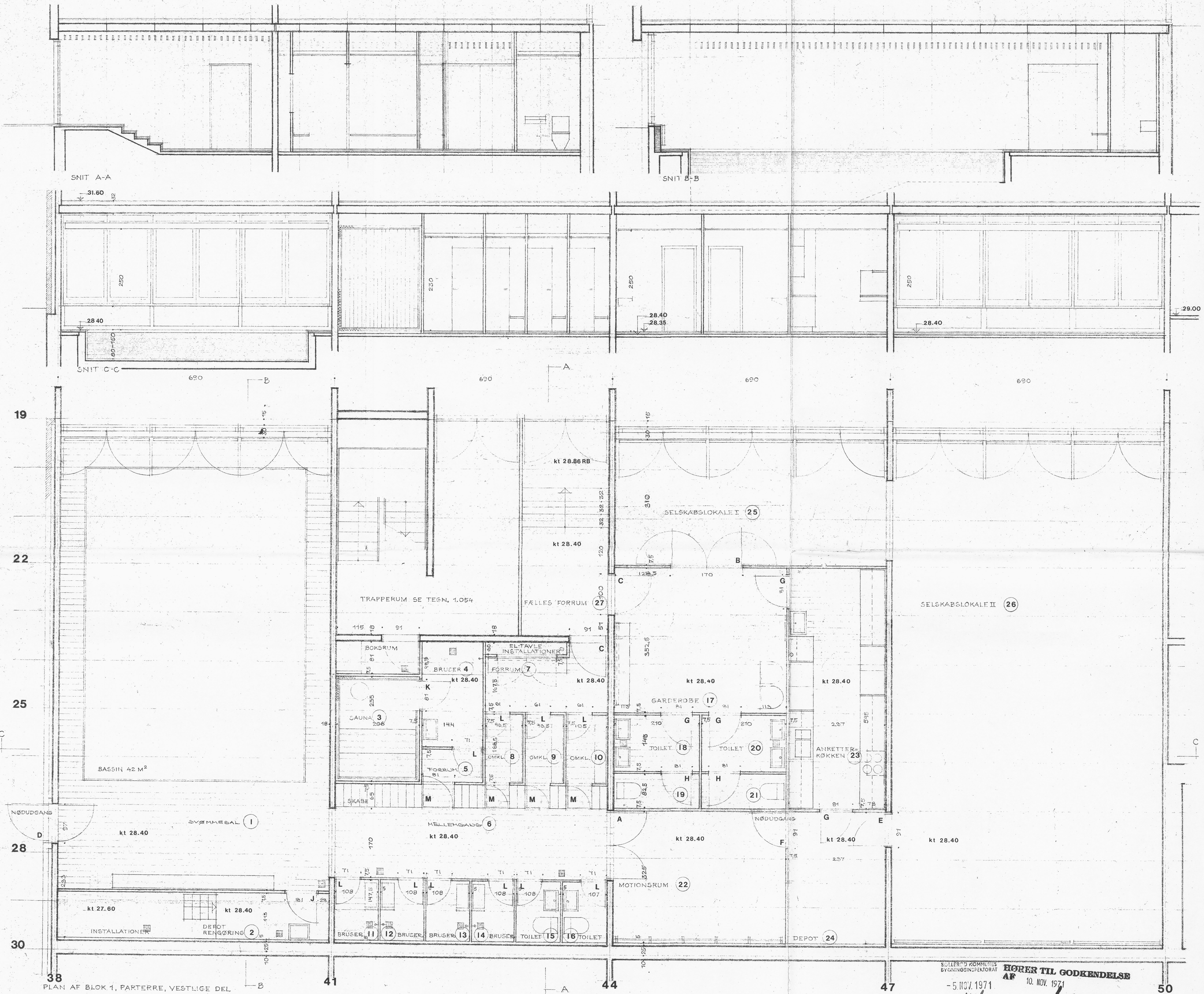
PLAN AF BLOK 1, PARTERRE, VESTLIGE DEL
